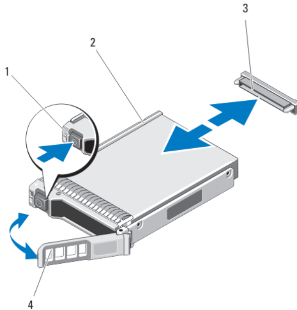
Figure 17. Retrait et installation d'un disque dur/SSD
