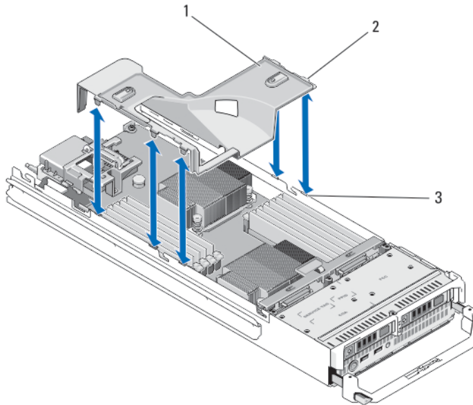
Figure 8. Retrait et installation d'un carénage de refroidissement
