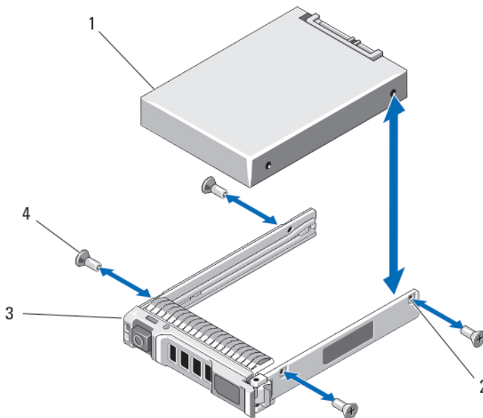
Figure 18. Retrait et installation d'un disque dur/SSD dans un support de disque dur
