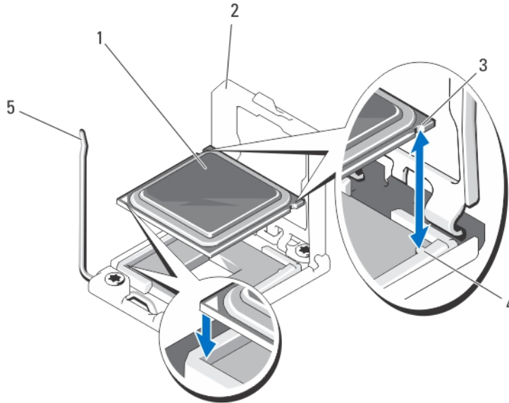
Figure 16. Retrait et installation d'un processeur
