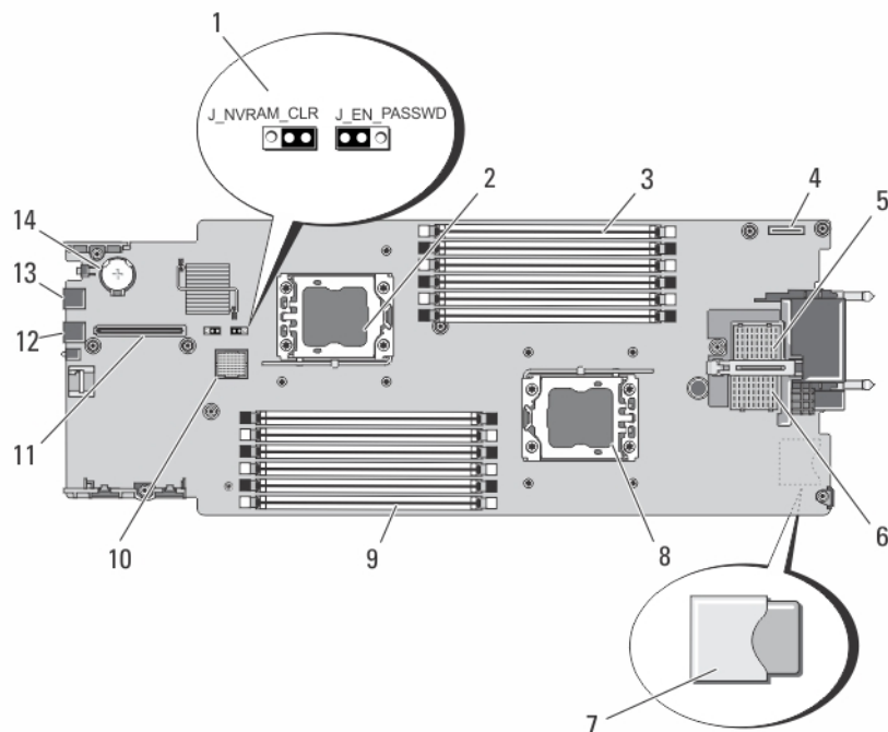
Figure 23. Connecteurs de la carte système
